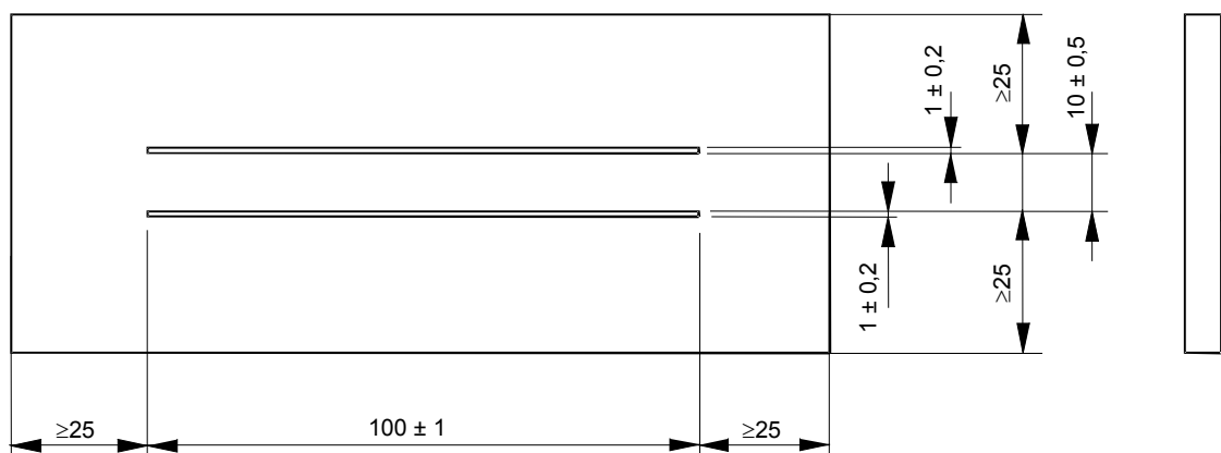
Figure 5 – Eprouvette avec électrodes peintes
