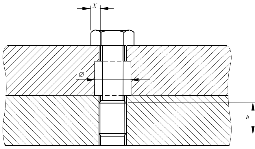
Figure 1 – Tolérances et espace pour fermetures filetées
