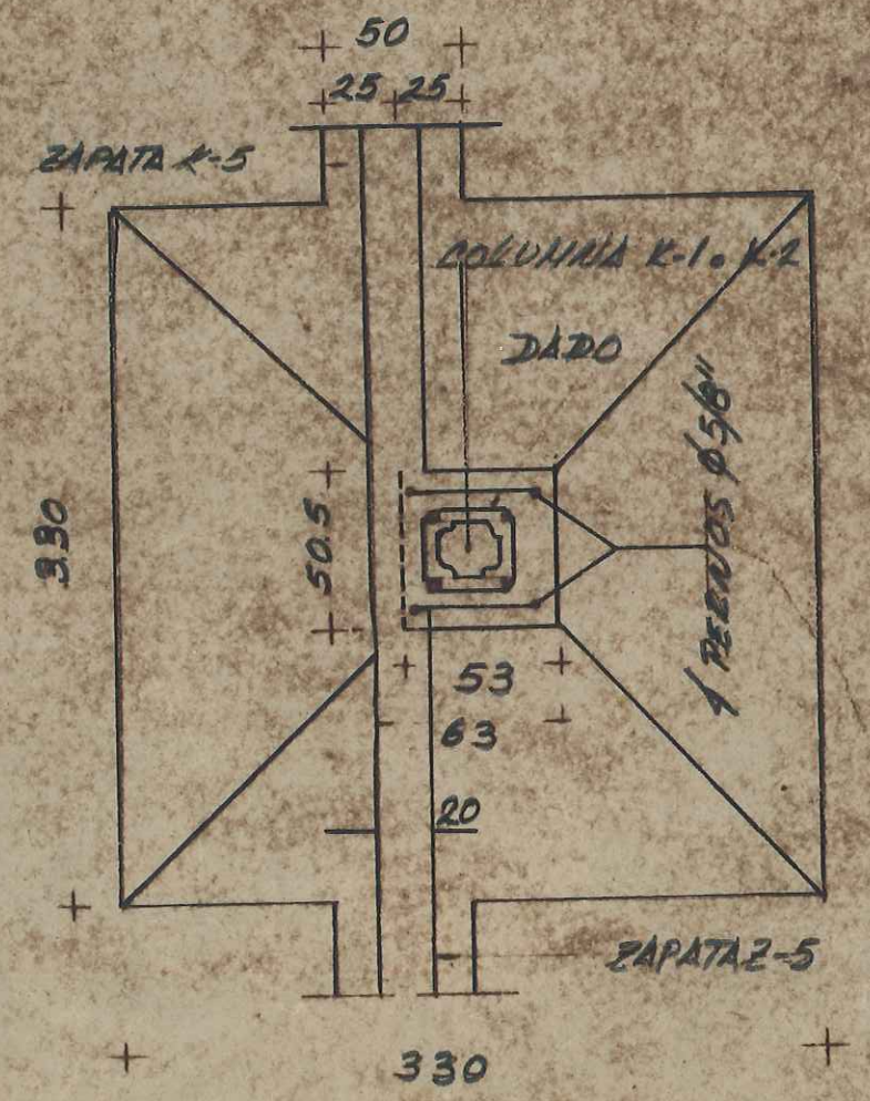
PLANTA ZAPATA Z-4 (ESC. 1:30)
