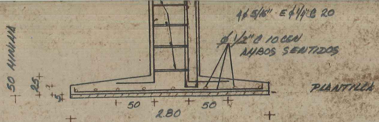
CORTE ELEV. ZAPATA Z-3
