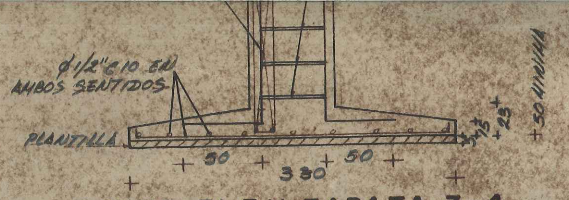
CORTE ELEV. ZAPATA Z-4
