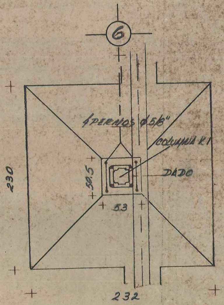
PLANTA ZAPATA Z-3 (ESC. 1:30)
